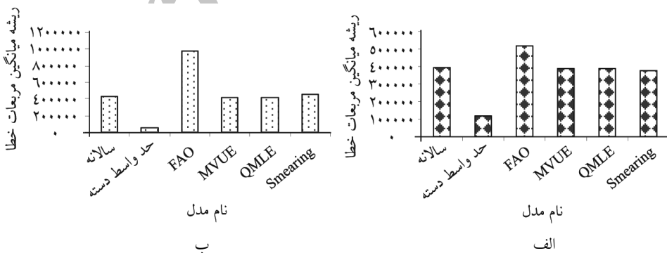
شکل ۴- هیستوگرام مقادیر شاخص آماری ریشه میانگین مربعات خطا (RMSE) برای مدل ۸۰-۲۰ (الف) و تمام داده‌ها (ب).
