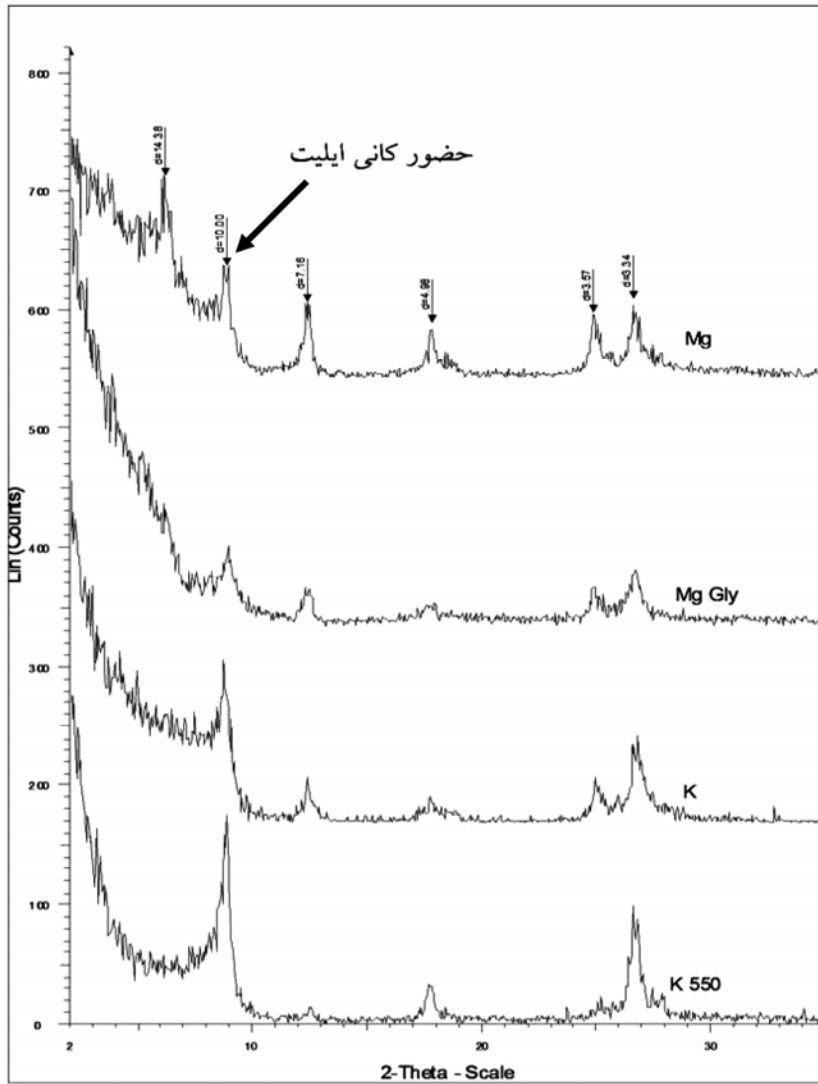
شکل ۲- پرتونگراشعه ایکس بخش رس، پیک 10^{\circ}A نشان دهنده کانی ایلیت می باشد (سری خاک مینودشت، افق B_{kl} ).
