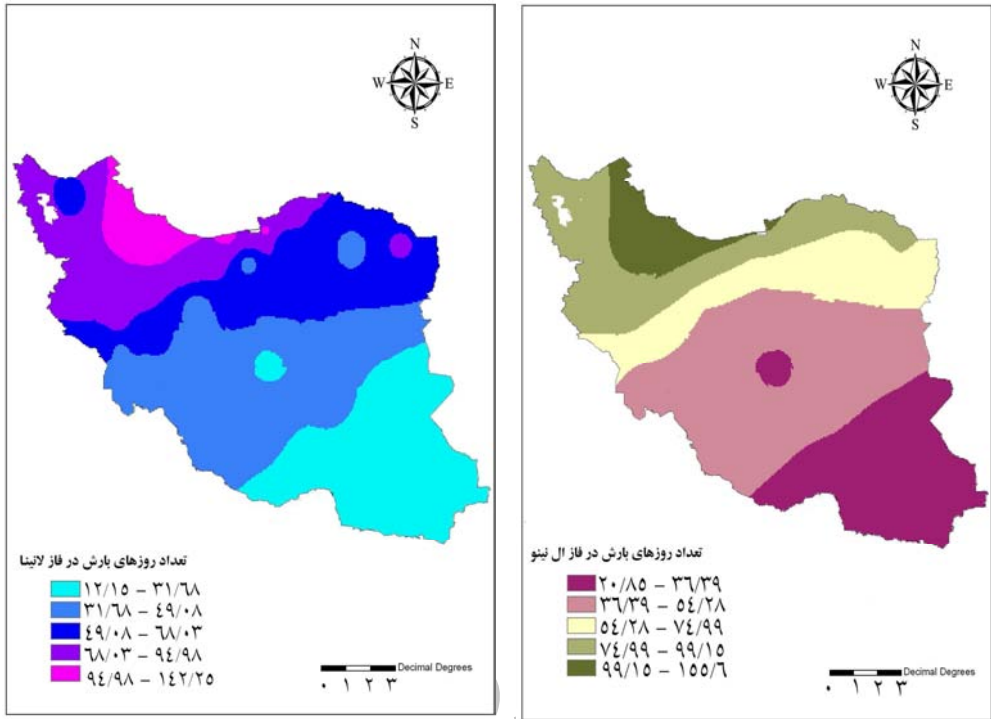
شکل ۳- پراکندگی تعداد روزهای بارانی در فازهای ال نینو و لائینا.
