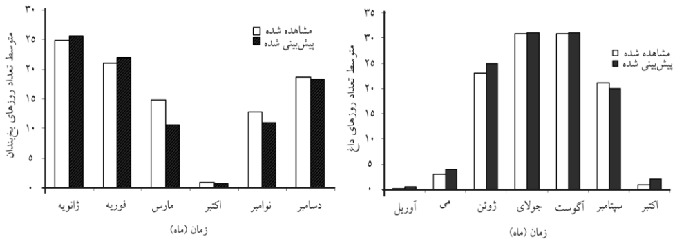
شکل 8- تعداد روزهای داغ و یخبندان مشاهده شده (1961-2229) و پیش‌بینی شده (2211-2232) در سنندج.
