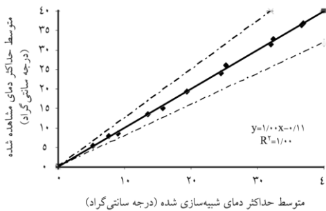
شکل 1- مقادیر مشاهده شده و شبیه‌سازی شده دمای حداکثر و حداقل در دوره آماری (1961-2229) در سنندج.
