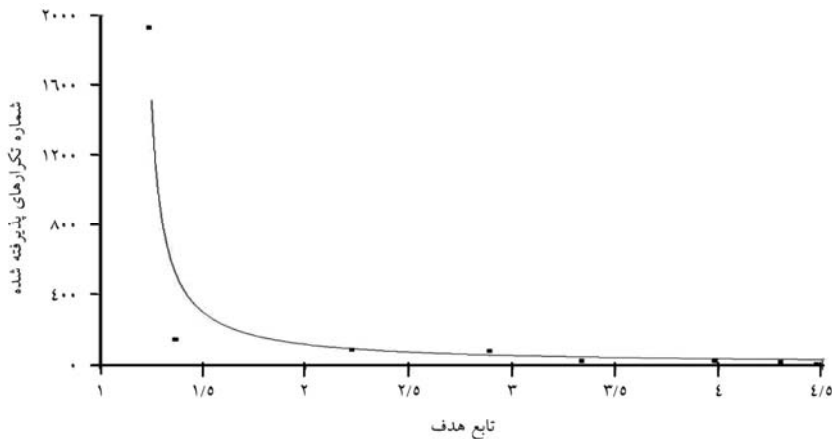
شکل ۴- منحنی y^{-1} = a + bx .
