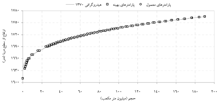
شکل ۳- توزیع رسوب در سد کرج در سال ۱۳۷۰.
