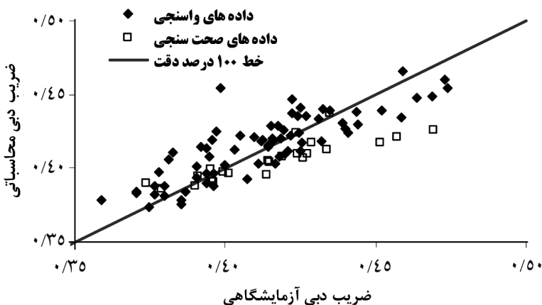
شکل ۴- مقایسه نتایج محاسباتی و آزمایشگاهی ضریب دبی سرریز جانبی مرکب برای داده‌های واسنجی و صحت‌سنجی.
