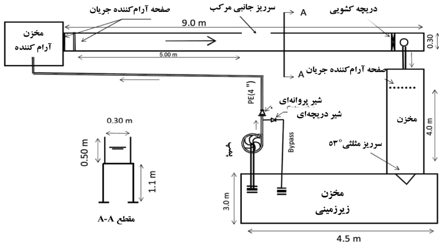
شکل ۲- نمای شماتیک کانال آزمایشگاهی.
