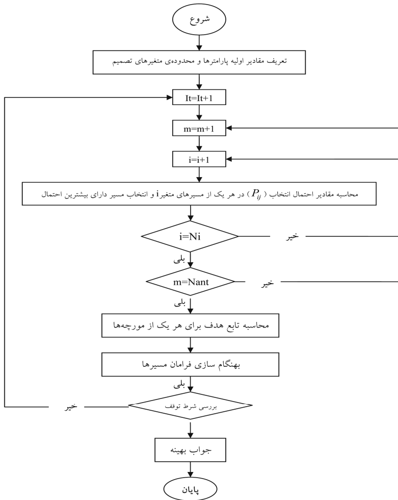
شکل ۲- نمودار گردش الگوریتم جامعه مورچه‌گان.
