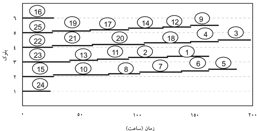
شکل ۹- نمودار زمان‌بندی تحویل بهینه آب به انشعابات.
