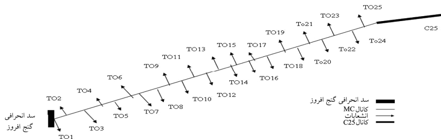
شکل ۳- شمای کلی کانال MC و انشعابات مربوطه.
