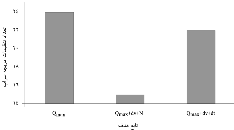
شکل ۸- مقادیر تعداد تنظیمات دریاچه سراب کانال در توابع هدف مختلف.
