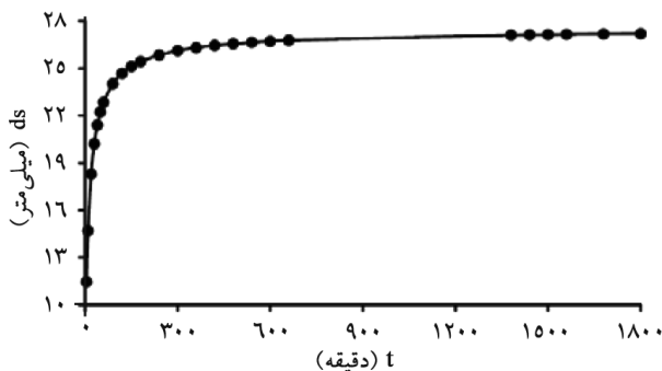
شکل ۱- توسعه زمانی عمق حفره آب‌شستگی.
