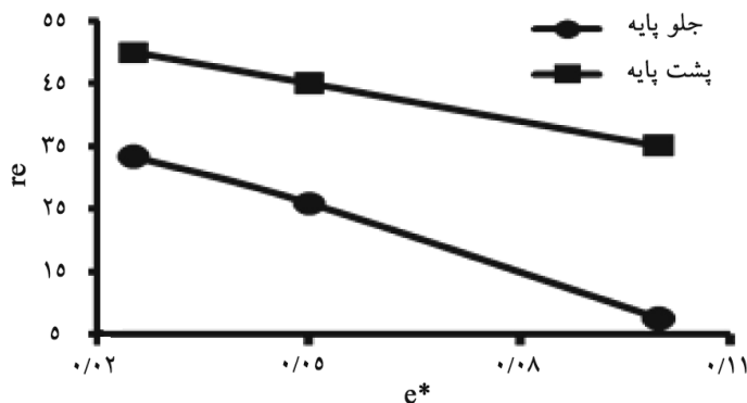
شکل ۲- درصد کاهش عمق حفره آبشستگی در جلو و پشت پایه پل (کانال II).
