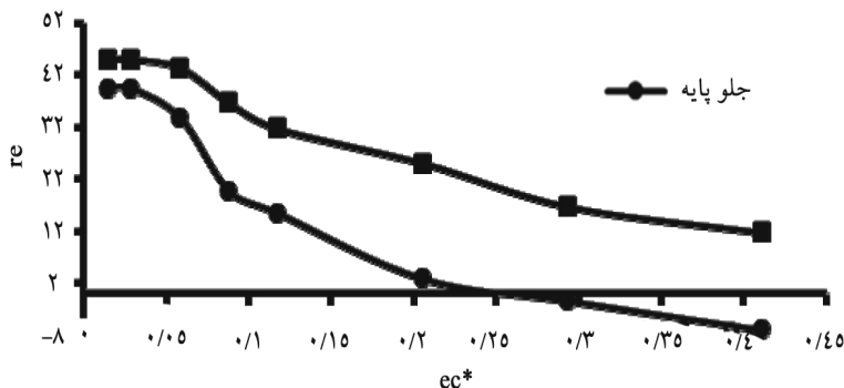
شکل ۳- درصد کاهش عمق حفره آب‌شستگی در جلو و پشت پایه پل (کانال II).
