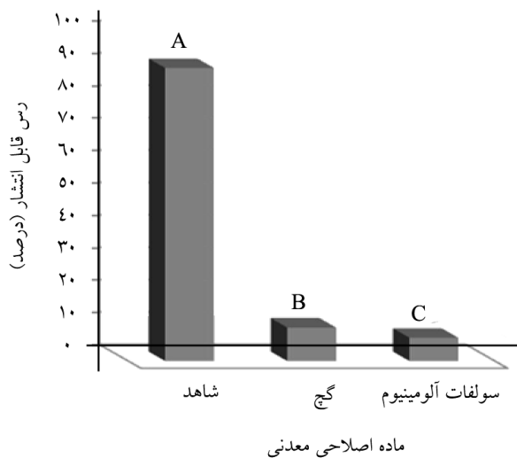
شکل ۱- تأثیر نوع ماده اصلاحی معدنی بر درصد رس قابل انتشار.
