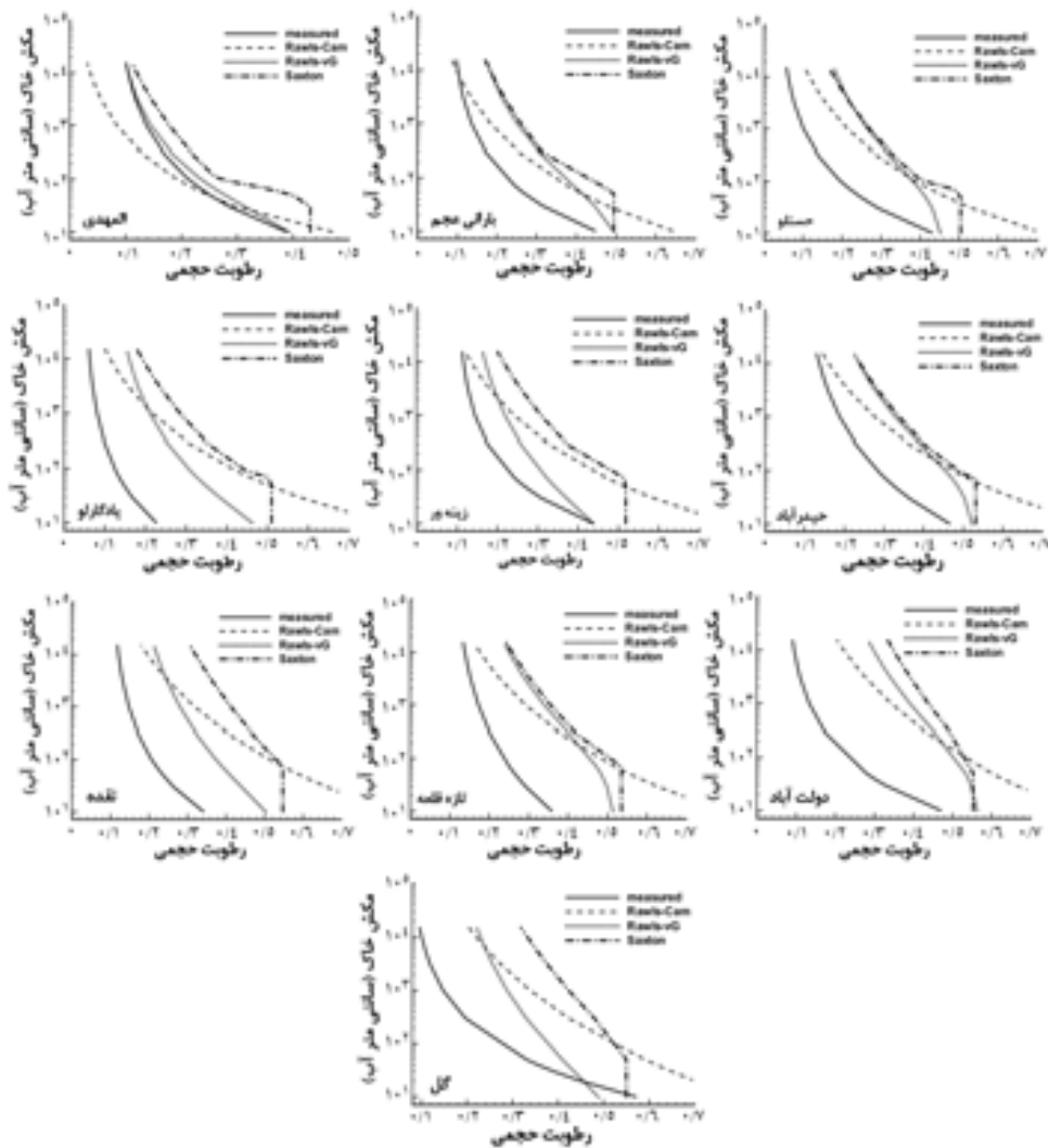
شکل ۲- منحنی مشخصه آب خاک اندازه‌گیری شده به روش صحرائی شانی و شبیه‌سازی شده توسط تابع انتقالی راولز و براکنسیک (۱۹۸۵) و سکستون و همکاران (۱۹۸۶) برای خاک‌های منطقه مورد مطالعه.
