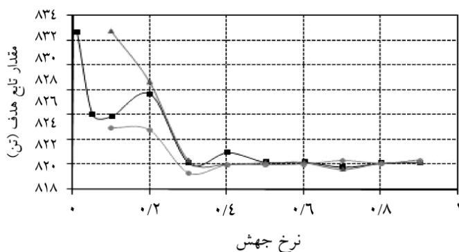
شکل ۵- نتایج ۳ مرحله آنالیز حساسیت نرخ جهش.
