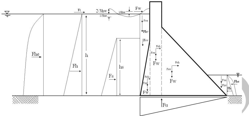
شکل ۱- نمایی از بارگذاری در نظر گرفته شده در مدل.
