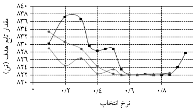
شکل ۶- نتایج ۳ مرحله آنالیز حساسیت نرخ انتخاب.
