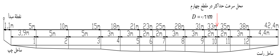
شکل ۳- جانمایی مقاطع عرضی انتخابی رودخانه پسیخان، مقاطع عمودی اندازه گیری نیم رخ سرعت و محل سرعت بيشترين در هر مقطع.
