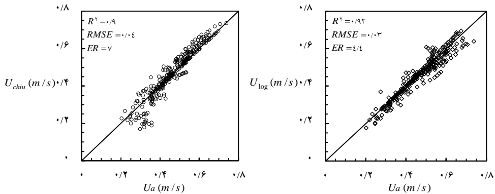
شکل ۷- نمودار سرعت نقطه‌ای محاسبه شده توسط روش چيو و لگاریتمی نسبت به مقادير اندازه‌گیری شده در کلیه مقطع انتخابی رودخانه پسیخان.
