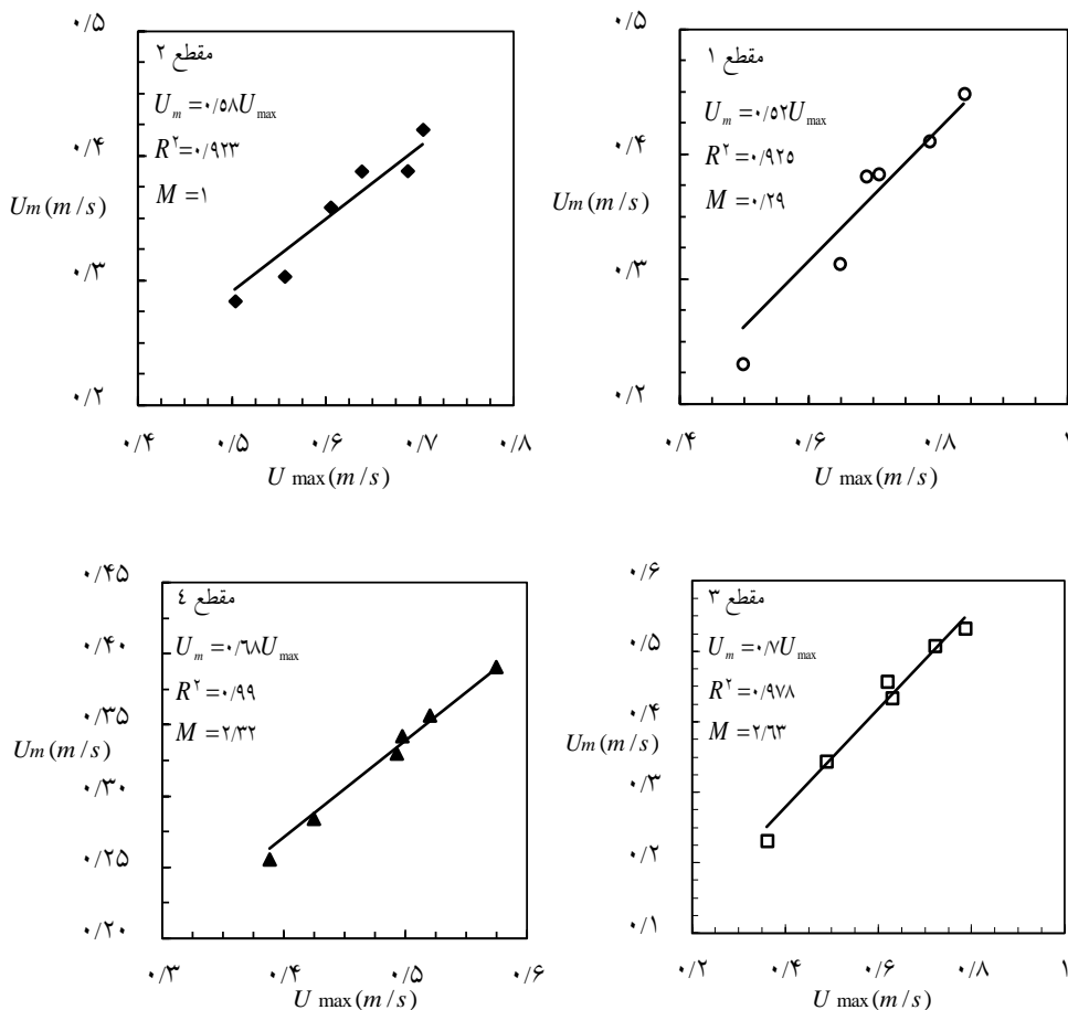
شکل ۵- نمودار سرعت متوسط- سرعت حداکثر برای ۴ مقطع انتخابی رودخانهٔ پسپخان.
