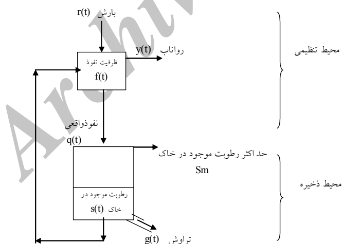
شکل ۷- نمودار شماتیک مدل نفوذپذیری دیسکن و نازیموف.
