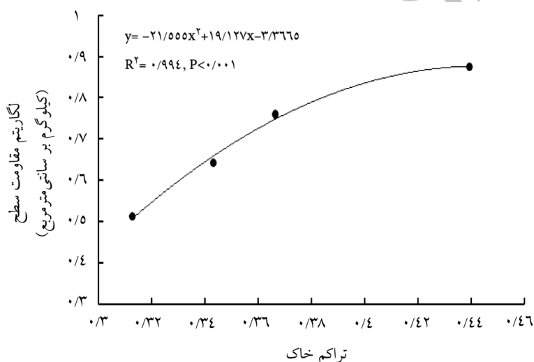
شکل ۳- رابطه بین مقاومت سطح و تراکم تحت تأثیر پلی‌وینیل استات در خاک مارنی.
