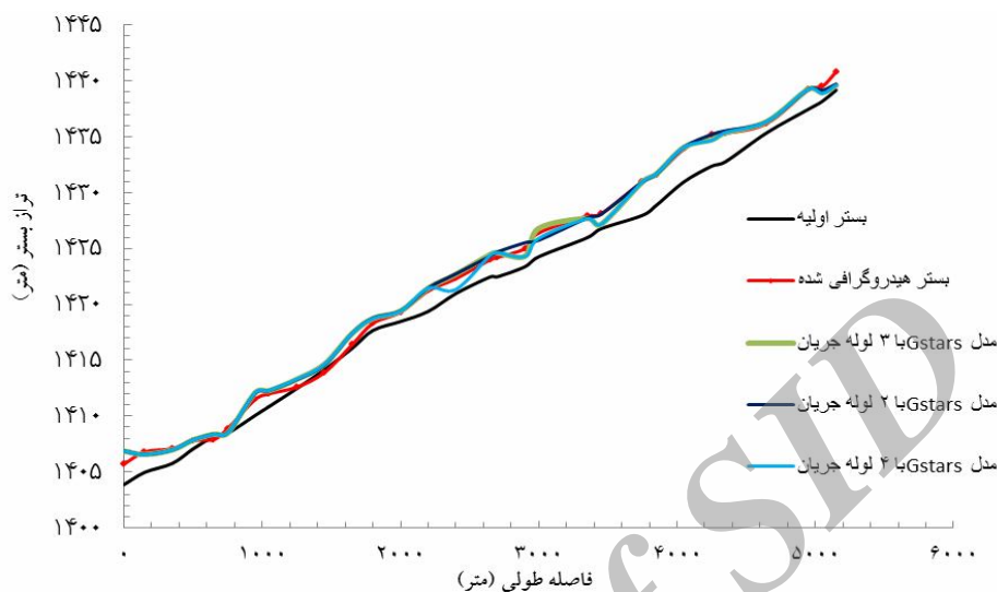
شکل ۴- نیمرخ خط القعر مخزن به‌ازای لوله‌های جریان مختلف.
