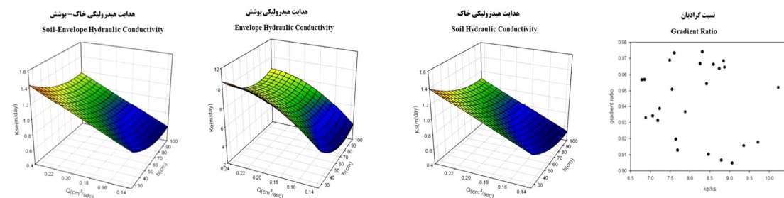
شکل ۳- مقادیر پیش‌بینی شده هدایت هیدرولیکی خاک- پوشش، هدایت هیدرولیکی پوشش، هدایت هیدرولیکی خاک و نسبت گرادیان در پوشش معدنی.
