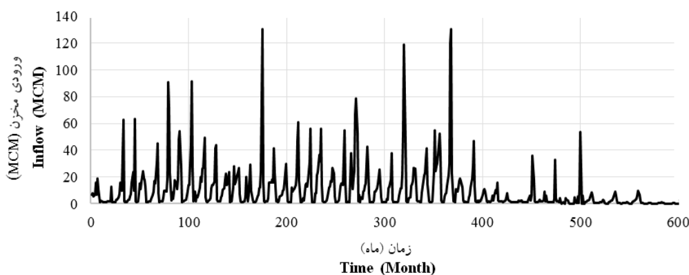
شکل ۱- تغییرات ماهانه ورودی به مخزن سد نهب بر حسب میلیون مترمکعب- مطالعات مصوب برنامه‌ریزی منابع آب سد نهب.
