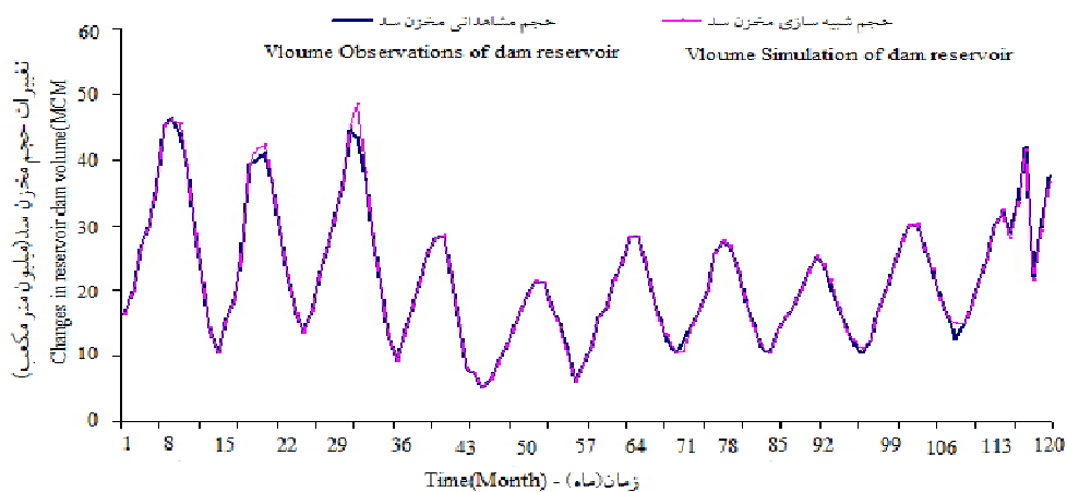
شکل ۴- مقایسه مقدار حجم مخزن مشاهده‌ای و شبیه‌سازی شده از مخزن سد.
