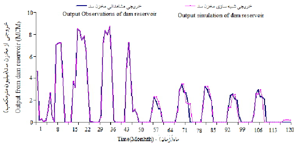
شکل ۳- مقایسه مقدار خروجی مشاهده‌ای و شبیه‌سازی شده از مخزن سد.
