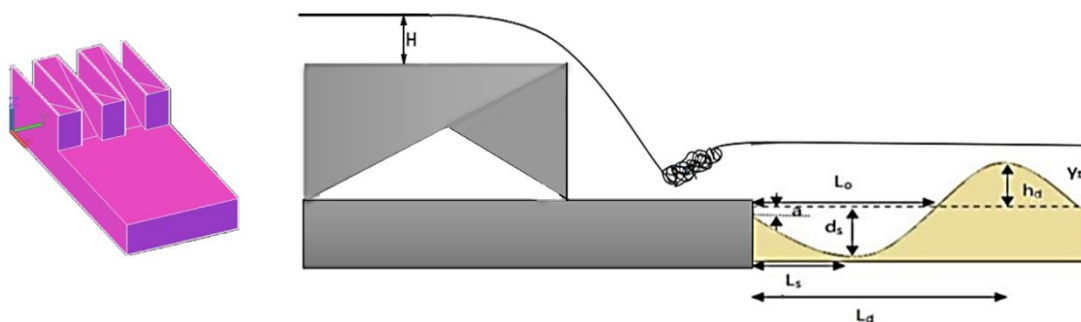
شکل ۲- طرح‌واره‌ای از سرریز کلید پیاپی با حفره آب‌شستگی و پارامترهای مشخصه آن.
