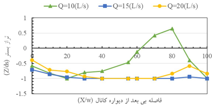
شکل ۷- پروفیل آب‌شستگی در عرض کانال در دبی‌های مختلف در سرریز ۹ کلیدی.
