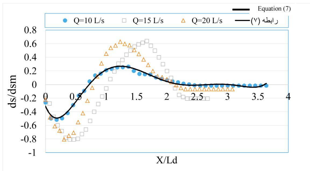
شکل ۱۰- پروفیل بی بعد آب شستگی در سرریز لبه تیز.
