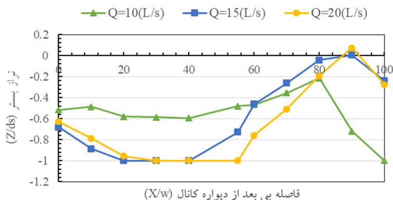
شکل ۶- پروفیل آب‌شستگی در عرض کانال در دبی‌های مختلف در سرریز ۵ کلیدی.
