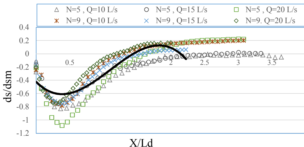
شکل ۹- پروفیل بی بعد آب شستگی در رسوبات غیر چسبنده.
