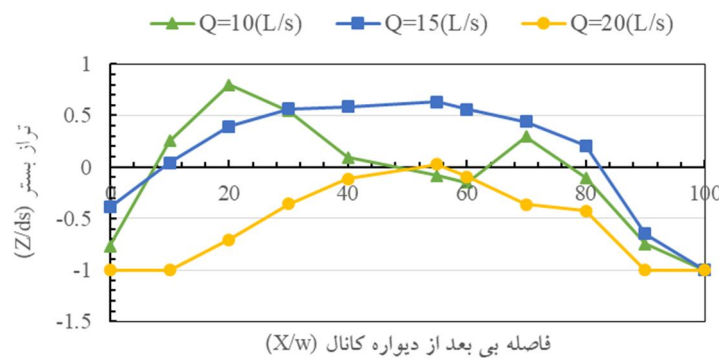
شکل ۸- پروفیل آب‌شستگی در عرض کانال در دبی‌های مختلف در سرریز لبه تیز (خطی).
