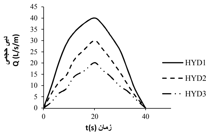
شکل ۴- هیدروگرافهای جریان ورودی به کانال.
