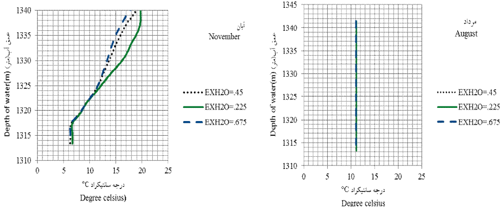
شکل ۴- تأثیر ضریب EXH2O در دوران لایه‌بندی مخزن. Figure 4. Effect of EXH2O in reservoir layering.
