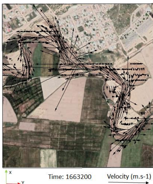
شکل ۶- بردارهای سرعت. Figure 6. Velocity vectors.
