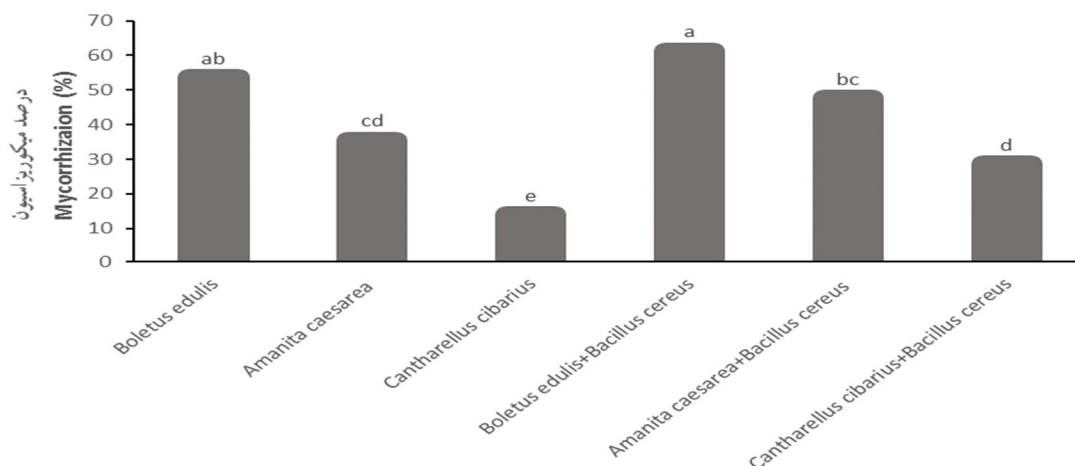
شکل ۲- نتایج مقایسه میانگین اثر قارچ‌های اکتومیکوریز بر درصد میکوریزاسیون کاج سیاه. میانگین‌های با حروف مشترک تفاوت معنی‌داری بر اساس آزمون LSD ندارند.
