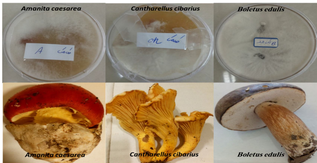
شکل ۱- میسلیم‌های رشد یافته در محیط کشت MMN. بالا: قارچ‌های اکتو میکوریز؛ پایین. Fig. 1.; grieved mycelium in MMN medium, Up; Ectomycorrhizal fungi, Down.
