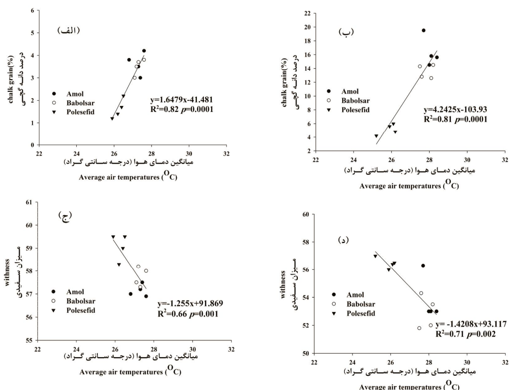
شکل ۳- رابطه بین درصد گچی دانه (طارم هاشمی (الف) و شیرودی (ب)) و میزان سفیدی (طارم هاشمی (ج) و شیرودی (د)) با میانگین دمای هوا در طول دوره پر شدن دانه برنج (از مرحله ۵۰ درصد گلدهی تا مرحله رسیدگی برداشت) اعداد در محور عمودی متفاوت می‌باشد.
