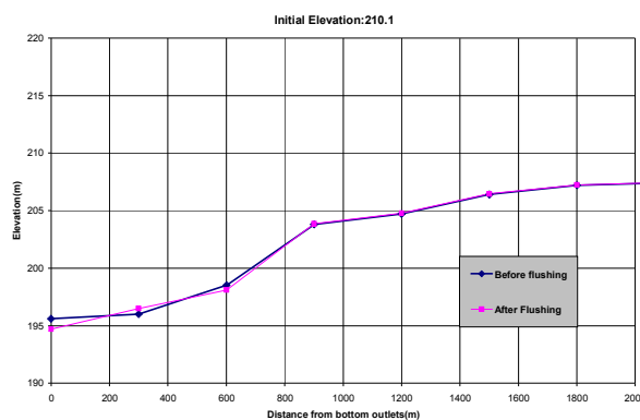
شکل ۵ پروفیل طولی قبل و بعد از انجام فلاشینگ با تراز ابتدایی ۲۱۰/۱ (تراز آبگیر نیروگاه)
