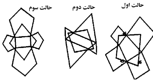
شکل ۱۲ تعمیم مسئله ۵
