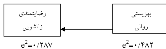
شکل ۳- مدل تحلیل مسیر
