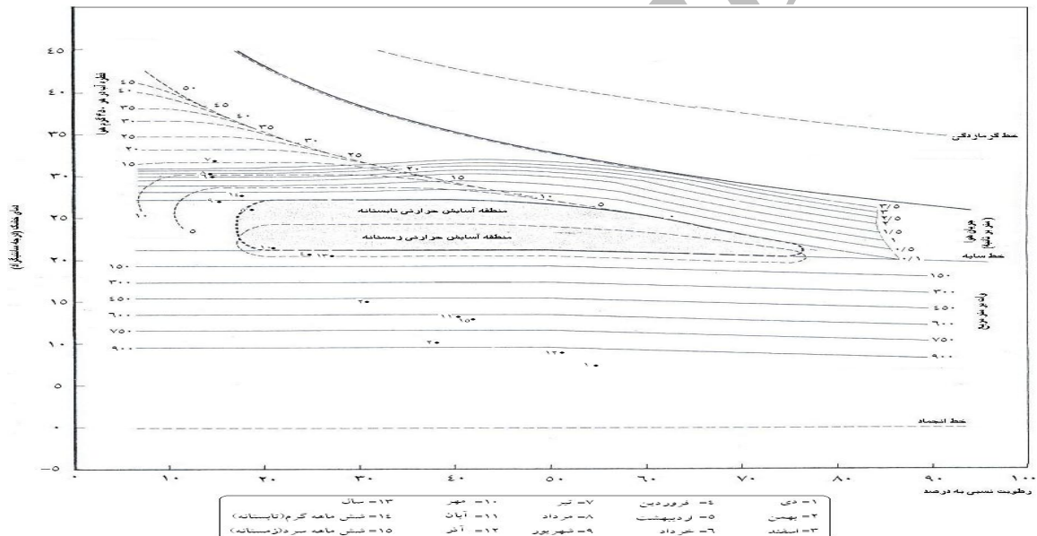
شکل ۳: نمودار زیست-اقلیمی اولگی (Olgay, 1973) وضعیت آسایش حرارتی ایستگاه یزد به تفکیک ماهانه
