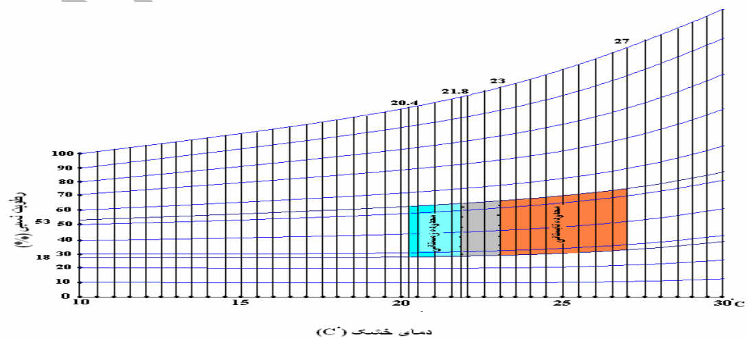
شکل ۴: جدول زیست-اقلیمی آسایش حرارتی در تابستان و زمستان برای شهر یزد
