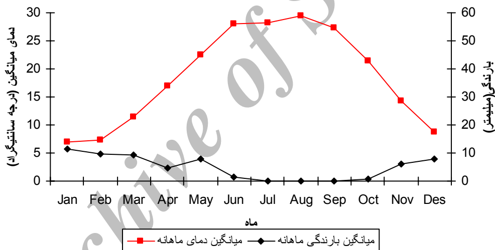
شکل ۲- کلیماگرام ایستگاه یزد طی سالهای ۱۹۹۷-۲۰۰۶
