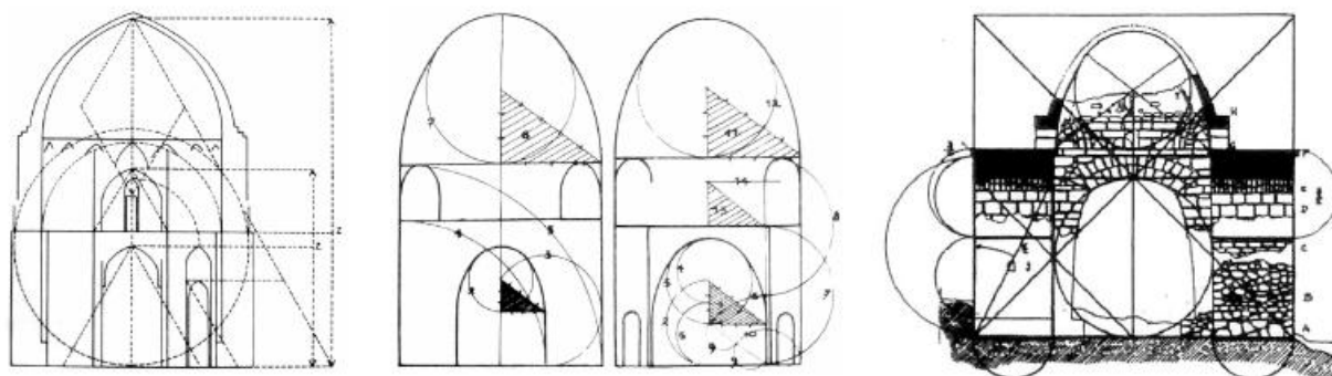
تصویر ۲- راست: تحلیل هندسی چهارتاقی نیاسراز هاردی. ماخذ: (گذار، ۱۳۸۸، ۱۵۳). وسط و چپ: تحلیل هندسی گنبد تاج الملک مسجد جامع اصفهان. ماخذ: (پوپ، ۱۳۶۵، ۲۳).
