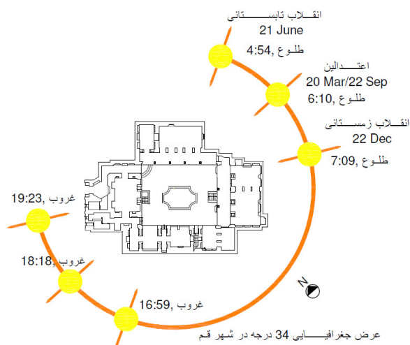
تصویر ۱- وضعیت تابش خورشید - خانه علیقلی خان زند. ماخذ: (اطلاعات تصویر www.geog.ubc.ca - مهندسی مشاور امکو).
