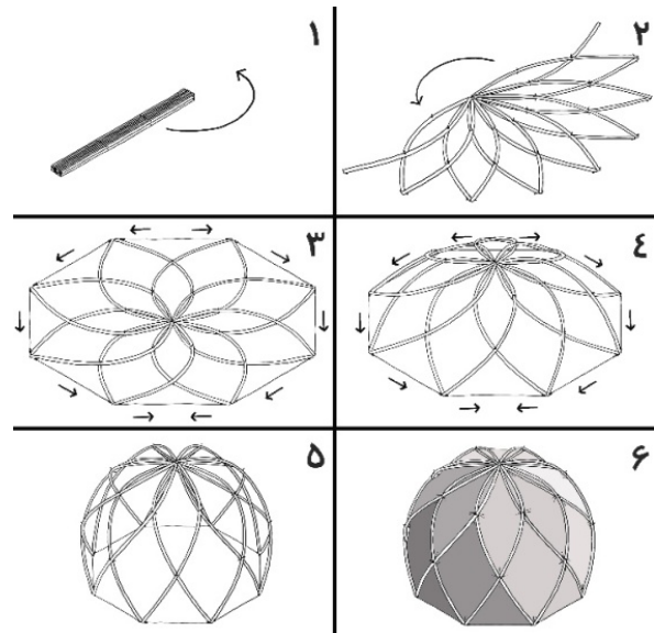
تصویر ۱۲- سایه بان‌های تغییرپذیر خم‌شو که به کمک مکانیزم ملهم از گل میمون باز و بسته می‌شوند.
