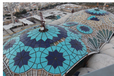
تصویر ۵- پوسته‌های گنبدی مجموعه مصلی اصفهان.
