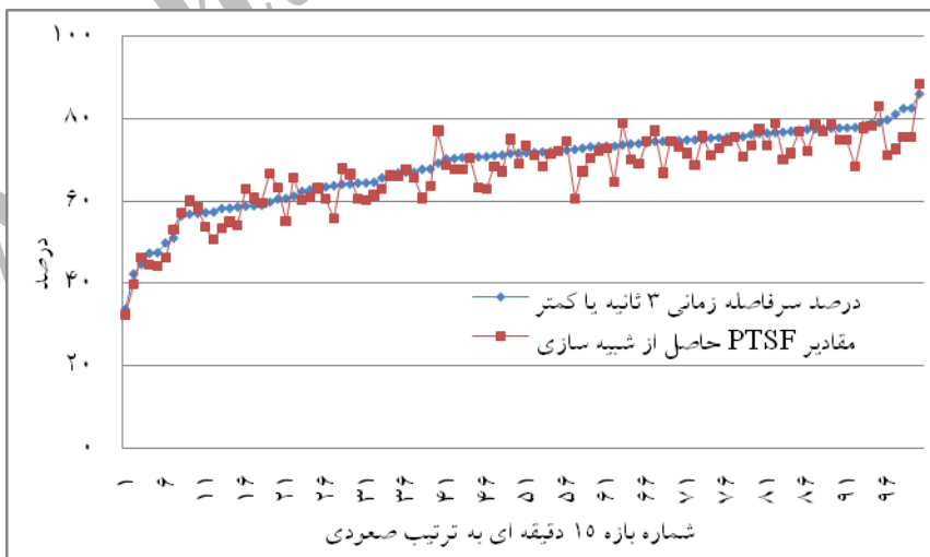
نمودار چهار: مقایسه درصد سرفاصله زمانی و PTSEF در بازه ۱۵ دقیقه‌ای، راه دوخطه قم - اسلامشهر
