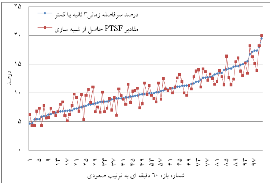
نمودار سه: مقایسه درصد سرفاصله زمانی و PTSEF در بازه ۶۰ دقیقه ای، راه دوخطه زنجان - میانه
