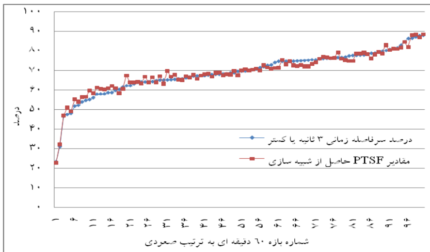
نمودار یک: مقایسه درصد سرفاصله زمانی و PTSD در بازه ۶۰ دقیقه‌ای، راه دوخطه قم - اسلامشهر
