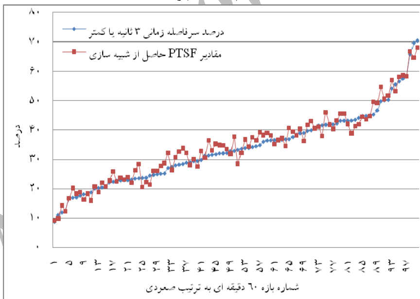
نمودار دو: مقایسه درصد سرفاصله زمانی و PTSD در بازه ۶۰ دقیقه‌ای، راه دوخطه کرج - چالوس
