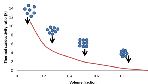
شکل ۲: اثر خوشه‌شدن و درصد حجمی بر روی ضریب هدایت حرارتی [۶]
