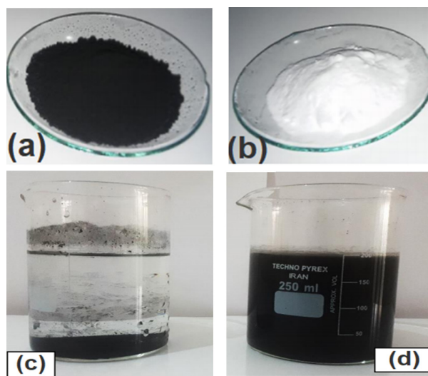
شکل ۶: (a) نانوکربن، (b) سدیم دودسیل سولفات، (c) نانوسیال کربن بدون سورفکتانت، (d) نانوسیال کربن با سورفکتانت [۱۳]
