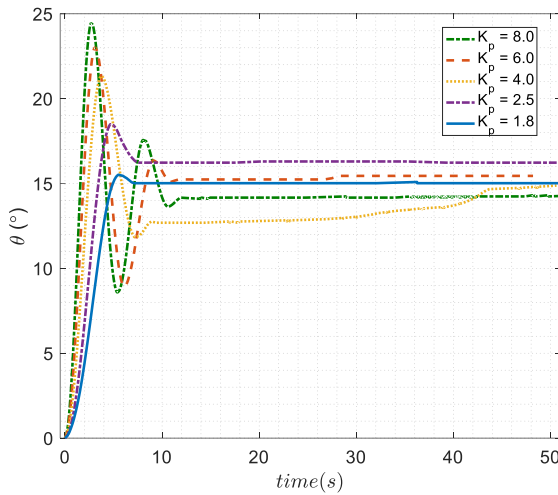
شکل ۱۰: دقت نشان‌دهنده‌ی محور اول به ازای تغییرات بهره تناسبی
