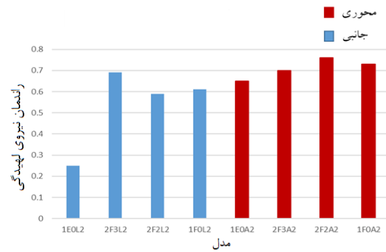
شکل ۲۵: نمودار راندمان نیروی لهیدگی عددی مدل‌های جانبی (فوم مقاوم و محوری).
