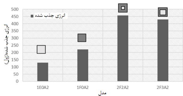
شکل ۱۴: نمودار انرژی جذب شده تعادلی ویژه نمونه‌ها در ۴/۹ میلی‌متر.
