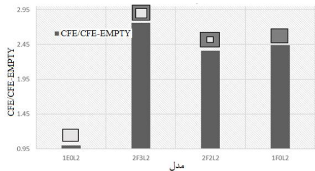
شکل ۲۶: نمودار نسبت راندمان نیروی لهیدگی مدل‌های جانبی با فوم مقاوم‌تر.
