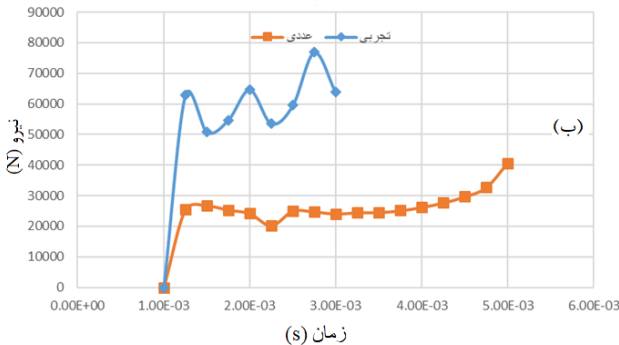
شکل ۱۲: الف) نمودار شتاب - زمان تجربی نمونه 1E0A2 (ب) نمودار نیرو - زمان تجربی و عددی نمونه 1E0A2.
