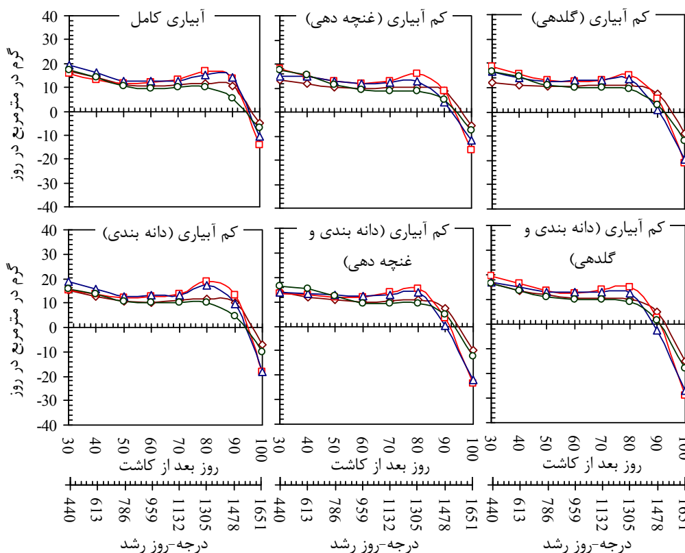
شکل ۳- روند تغییرات سرعت جذب خالص در اندام هوایی (گرم در مترمربع در روز) با روزه‌های بعد از کاشت و درجه-روز رشد در تیمارهای مختلف آبیاری و ارقام آفتابگردان (آذرگل: \diamond ، آلستار: \square ، آلیسون: \triangle و یوروفلور: \circ ).
