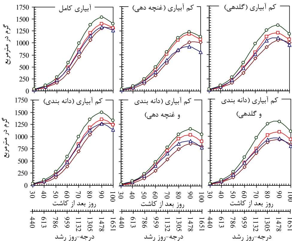
شکل ۵- روند تغییرات تجمع ماده خشک در اندام هوایی (گرم در مترمربع) با روزهای بعد از کاشت و درجه-روز رشد در تیمارهای مختلف آبیاری و ارقام آفتابگردان (آذرگل: \diamond ، آلیسون: \triangle ، الستار: \square ، آلیسون: \triangle ، و یوروفلور: \circ ).
