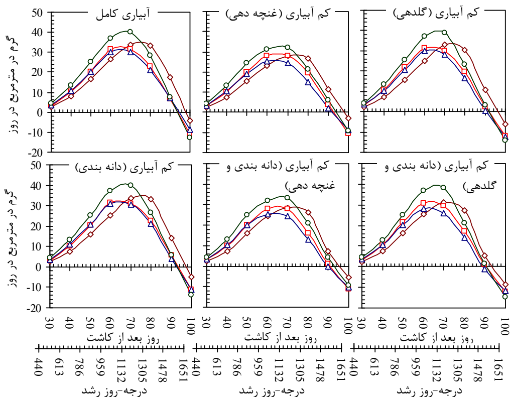
شکل ۲- روند تغییرات سرعت رشد محصول در اندام هوایی (گرم در مترمربع در روز) با روزهای بعد از کاشت و درجه-روز رشد در تیمارهای مختلف آبیاری و ارقام آفتابگردان (آذرگل: \diamond ، آلستار: \square ، آلیسون: \triangle و یوروفلور: \circ ).
