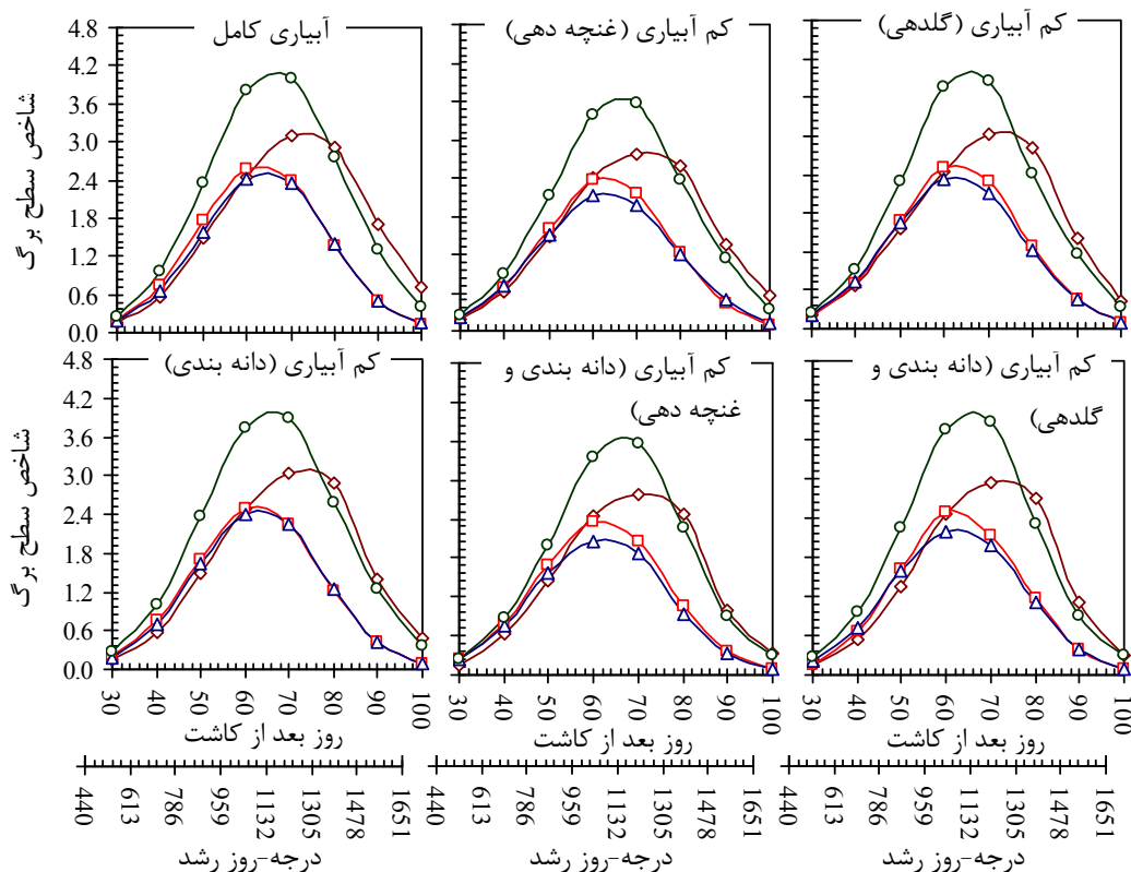
شکل ۱- روند تغییرات شاخص سطح برگ با روزهای بعد از کاشت و درجه-روز رشد در تیمارهای مختلف آبیاری و ارقام آفتابگردان (آدرگل: \blacklozenge ، آلستار: \blacksquare ، آلیسون: \blacktriangle و یوروفلور: \bullet ).
