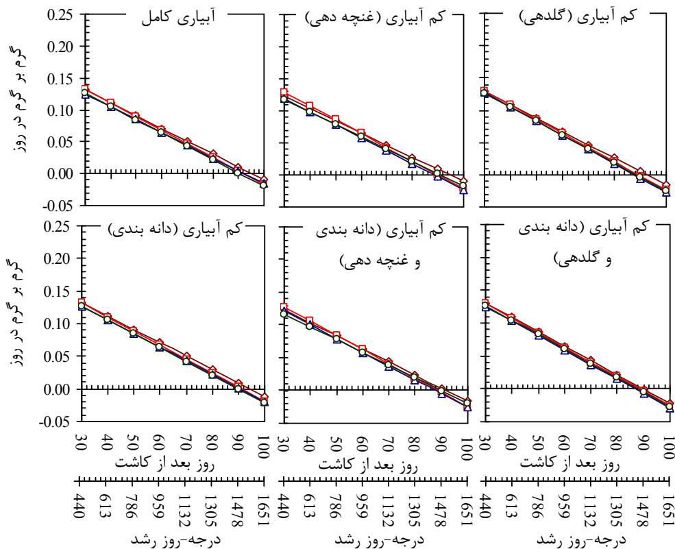
شکل ۴- روند تغییرات سرعت رشد نسبی در اندام هوایی (گرم بر گرم در روز) با روزهای بعد از کاشت و درجه-روز رشد در تیمارهای مختلف آبیاری و ارقام آفتابگردان (آذرگل: \blacklozenge ، آلستار: \blacksquare ، آلیسون: \blacktriangle و یوروفلور: \bullet ).
