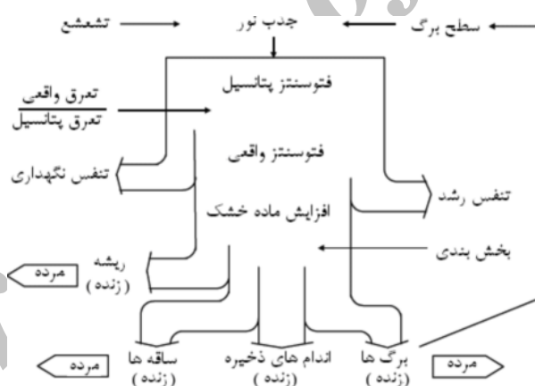
شکل ۱- مراحل شبیه‌سازی رشد گیاه با استفاده از مدل WOFOST (Supit et al., 1994)
