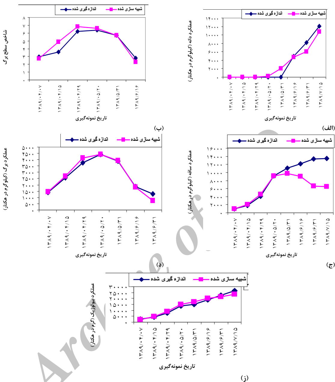
شکل ۳- مقایسه داده‌های شبیه‌سازی شده با داده‌های اندازه‌گیری شده در تولید ذرت دانه‌ای
