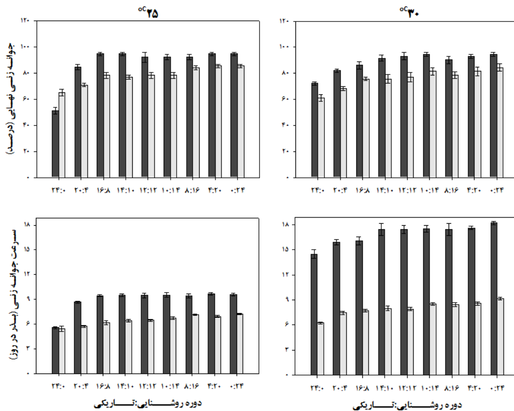
شکل ۳. اثر دوره روشنایی بر درصد نهایی و سرعت جوانه‌زنی در سوروف ( E. crus-galli ) و سوروف آبی ( E. oryzoides ) در دماهای ۲۵ و ۳۰ درجه سانتی‌گراد، طی هفت روز قرارگرفتن بذرها در شرایط جوانه‌زنی. خطوط عمودی (خطوط بار) نشان‌دهنده خطای استاندارد میانگین‌ها هستند.
