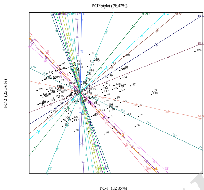
شکل ۲. نمودار دوجهی رگه × صفت بر پایه نخستین و دومین مؤلفه اصلی در رگه‌های برنج در شرایط تنش خشکی Figure 2. Biplot for line × trait in rice lines according to first and second principal components under drought stress.
