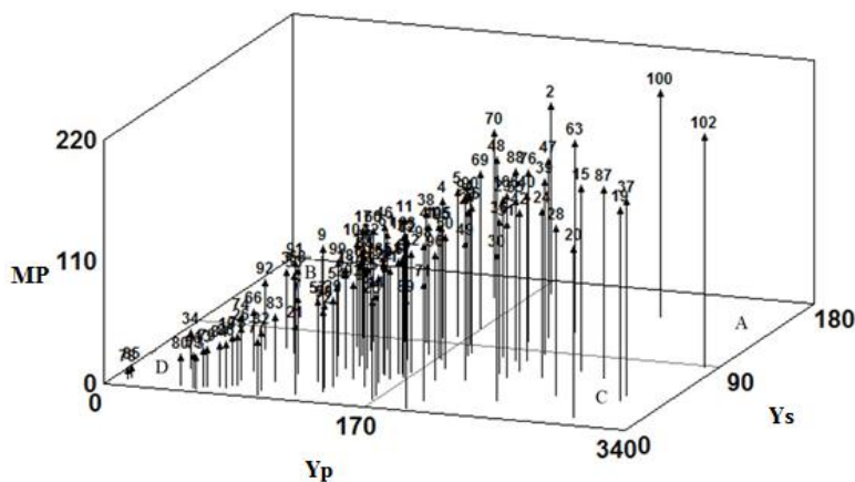
شکل ۱- نمودار تعیین ژنوتیپ‌های مقاوم به خشکی، بر اساس عملکرد آبی (Yp)، عملکرد دیم (Ys) و شاخص MP
