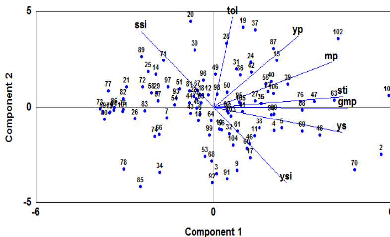
شکل ۲- نمایش بای پلات ۱۰۲ ژنوتیپ لوبیا در هشت شاخص تحمل به خشکی، بر اساس دو مؤلفه اول و دوم
