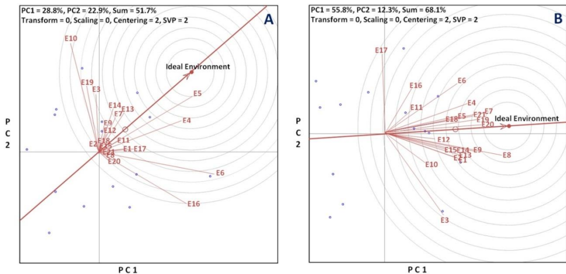
شکل ۲. نمایش نگاره‌ای GGE بای پلات روابط و "توانایی تفکیک بین ژنوتیپها و نمایندگی بودن" محیطها برای عملکرد دانه (A) و میزان روغن دانه (B) بر اساس ۲۱ محیط دیم (E1-E21)
