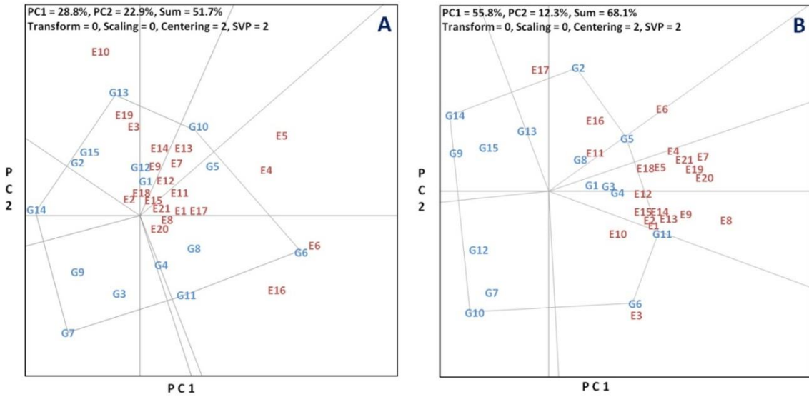
شکل ۱- الگو چندضلعی GGE بای پلات "کدام - برتر - کجا" برای عملکرد دانه (A) و میزان روغن دانه (B) بر اساس ۱۵ ژنوتیپ گلرنگ (G1-G15) ارزیابی شده در ۲۱ محیط دیم (E1-E21)
