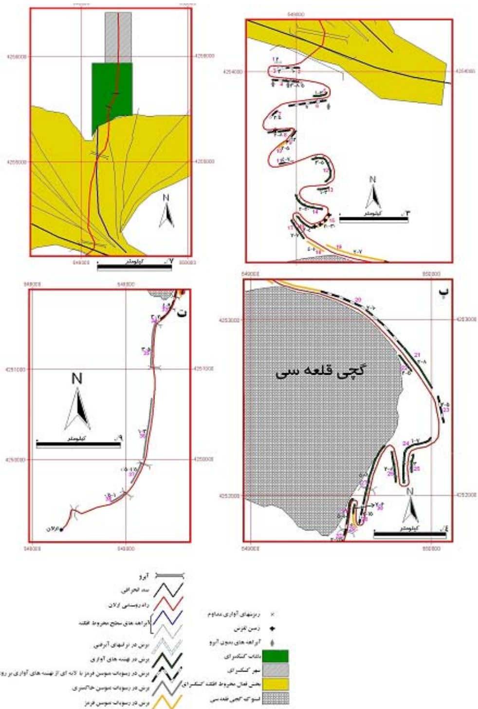
شکل شماره ۱۲ نقشه ریز پهنه‌بندی ویژگی‌های ژئومورفیک طول مسیر راه ارلان در واحد میوسن قرمز (الف)، واحد مخروط‌افکنه (ب)، واحد دره طوق مانند (پ)، و واحد فلات مرتفع (ت)
