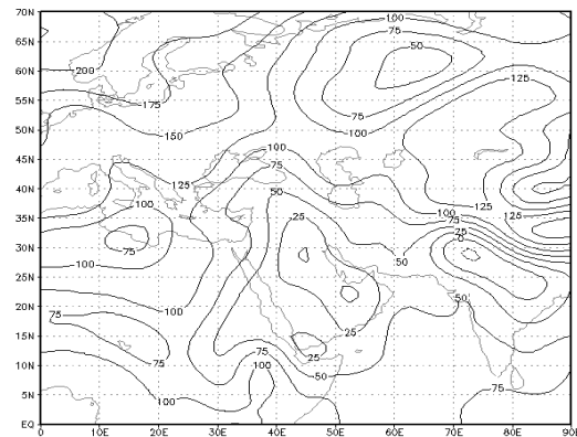
ل) روز هشتم. سطح ۱۰۰۰ هکتوپاسکال
