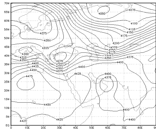
ز) روز هفتم. سطح ۶۰۰ هکتوپاسکال
