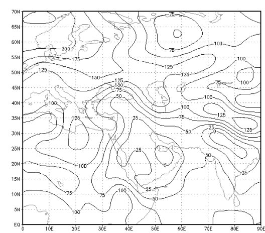
ه) روز هفتم. سطح ۱۰۰۰ هکتوپاسکال
