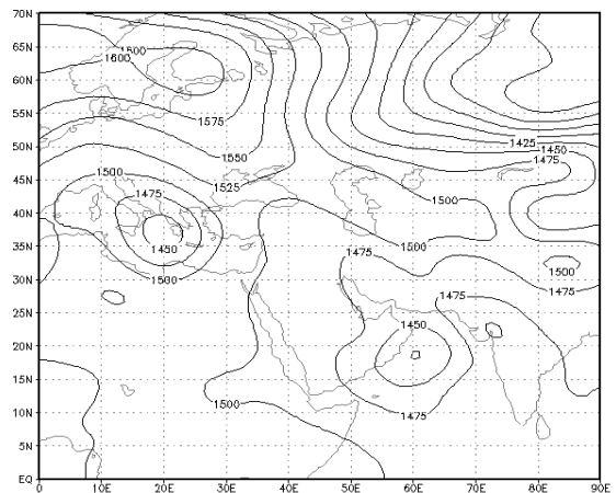
و) روز پنجم. سطح ۸۵۰ هکتوپاسکال
