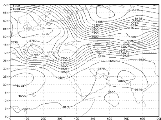
ص) روز هشتم. سطح ۵۰۰ هکتوپاسکال
