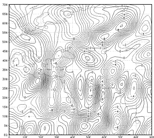
(و) روز هشتم سطح ۸۵۰ هکتوپاسکال
