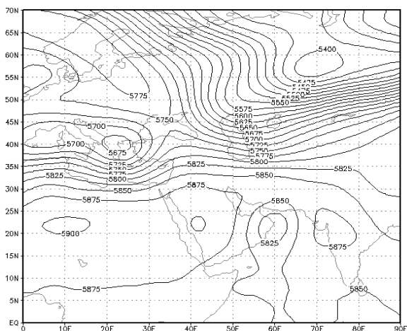
د) روز هشتم. سطح ۵۰۰ هکتوپاسکال
