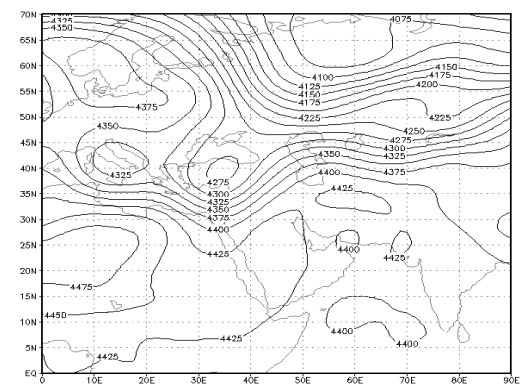
ن) روز هشتم. سطح ۶۰۰ هکتوپاسکال
