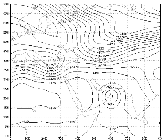
ج) روز هفتم. سطح ۶۰۰ هکتوپاسکال
