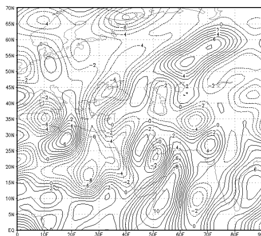
(ه) روز هشتم سطح ۱۰۰۰ هکتوپاسکال
