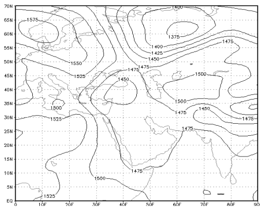
م) روز هشتم. سطح ۸۵۰ هکتوپاسکال
