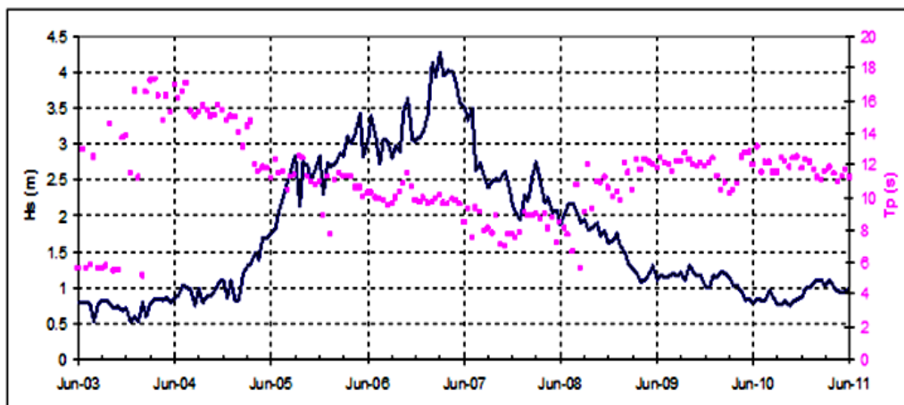
شکل ۲) ارتفاع امواج در سواحل چابهار ( http://hurricane.methaz.org/gonu/idamage.png )
