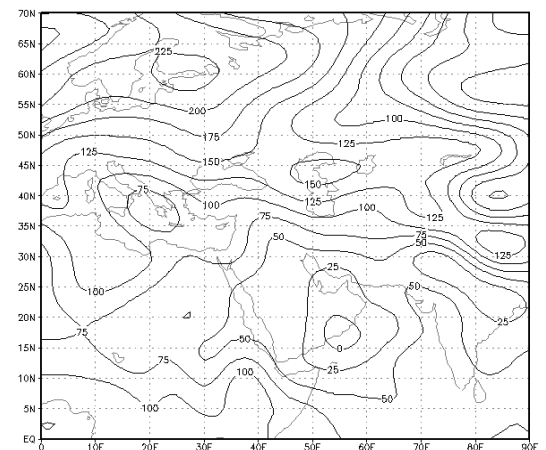
ه) روز پنجم. سطح ۱۰۰۰ هکتوپاسکال
