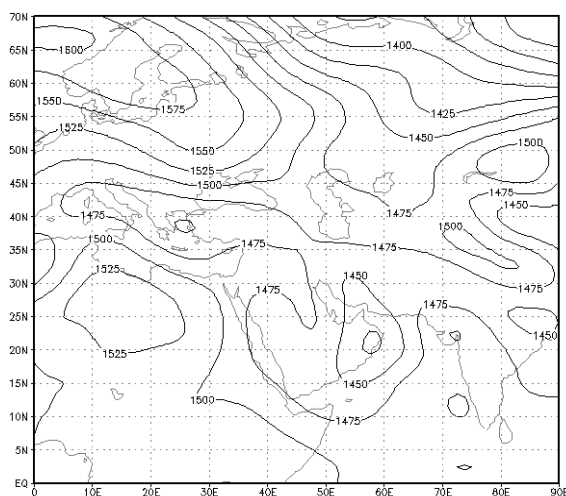
ب) روز ششم. سطح ۸۵۰ هکتوپاسکال
