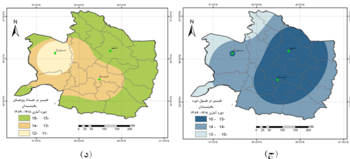
ادامه شکل ۳- پهنه‌بندی میزان تغییرات (ج) طول دوره یخبندان و (د) تعداد روزهای همراه با یخبندان در دوره اقلیمی آینده (۱۴۱۸-۱۳۸۹)
