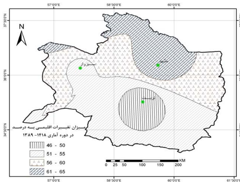
شکل ۶- پهنه‌بندی میزان تغییرات اقلیمی خراسان رضوی برای دوره اقلیمی آینده (۱۳۸۹-۱۴۱۸)
