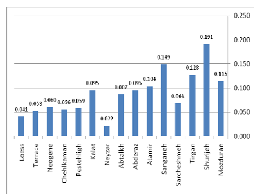
نمودار ۴- تمرکز تعداد چشمه‌ها به تفکیک سازندهای
