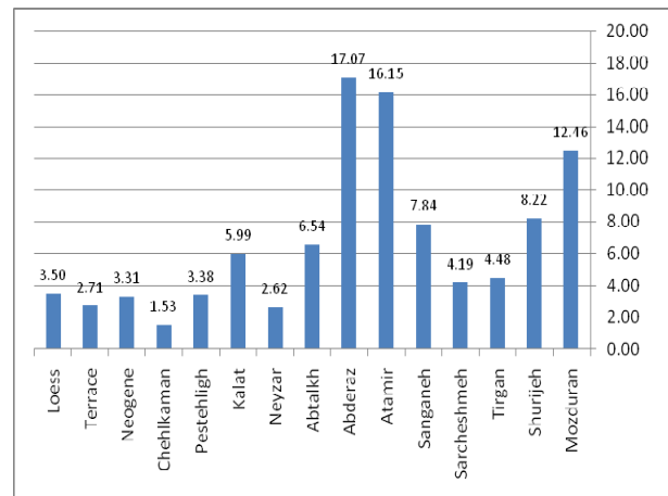
نمودار ۱- درصد گسترش سازندهای زمین شناسی در شهرستان کلان
