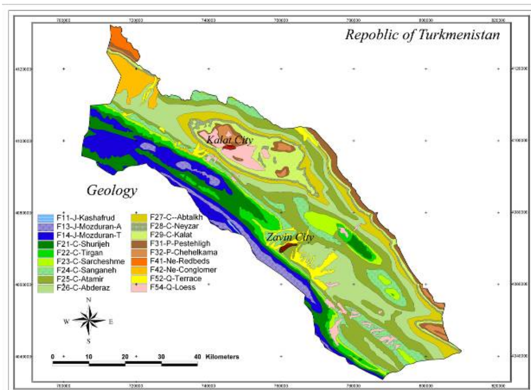
شکل ۵- نقشه زمین‌شناسی منطقه کلات
