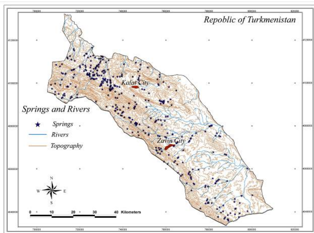
شکل ۶- نقشه پراکنش چشمه‌ها و رودخانه‌ها منطقه کلات
