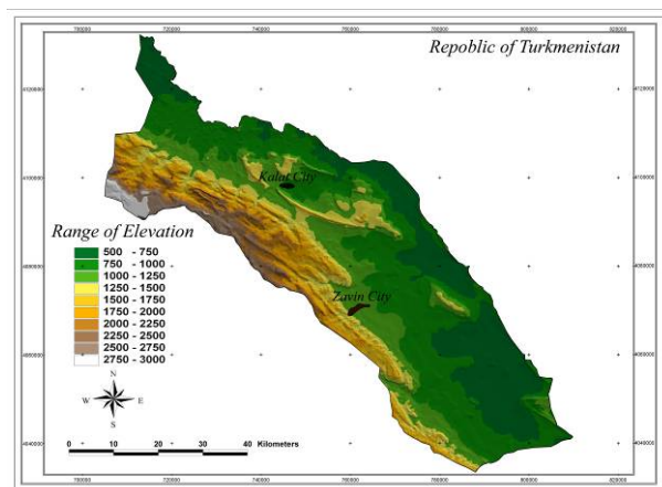
شکل ۳- طبقات ارتفاعی منطقه مطالعاتی
