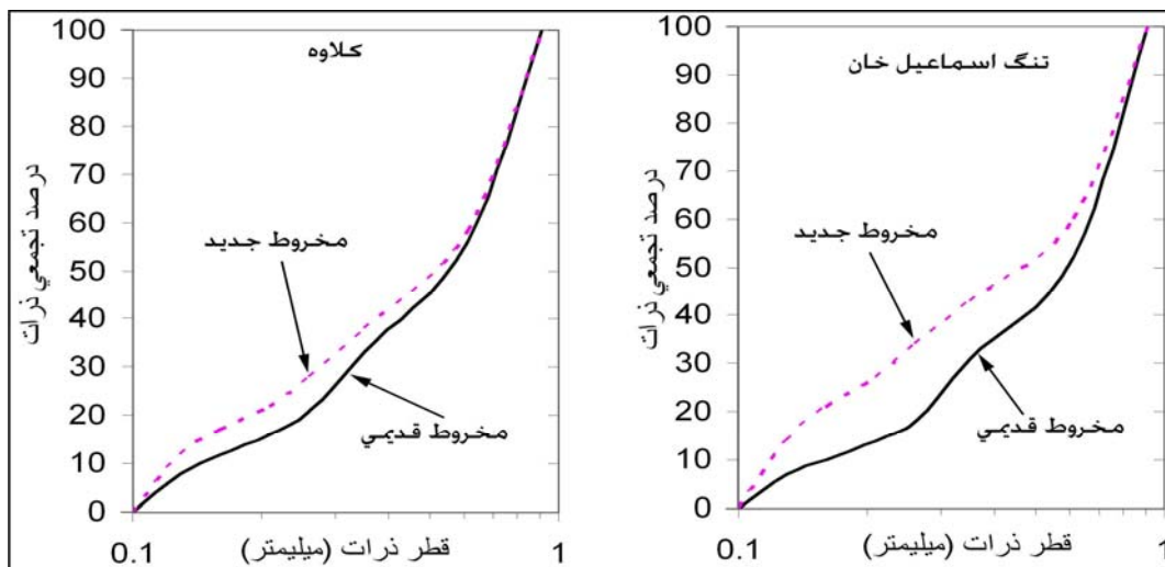
شکل ۸- منحنی درصد تجمعی رسوبات در مخروط افکنه‌های جدید و قدیمی روستاهای تنگ اسماعیل خان و کلاوه
