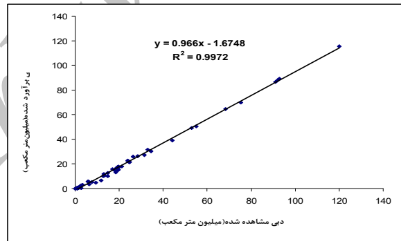
شکل شماره ۹: معادله‌ی رگرسیونی بین رواناب واقعی و برآورد شده با مدل شبکه‌ی عصبی مصنوعی
