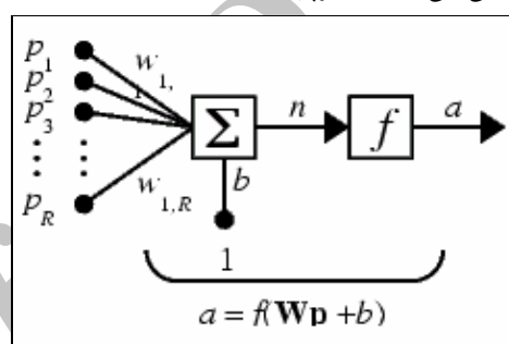
شکل شماره‌ی ۲: یک شبکه‌ی عصبی بسیار ساده
