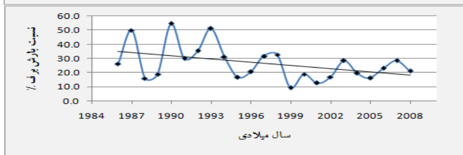
شکل ۹: نمودارهای روند میانگین دمای سالانه و نسبت بارش برف به بارش کل در ایستگاه اهر
