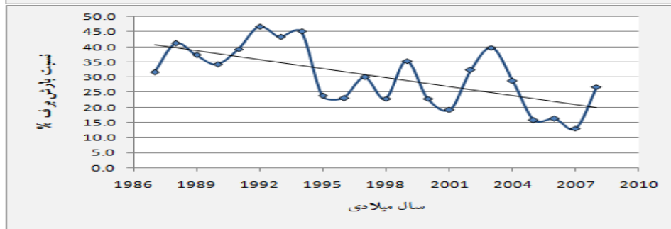
شکل ۸: نمودارهای روند میانگین دمای سالانه و نسبت بارش برف به بارش کل در ایستگاه خلخال
