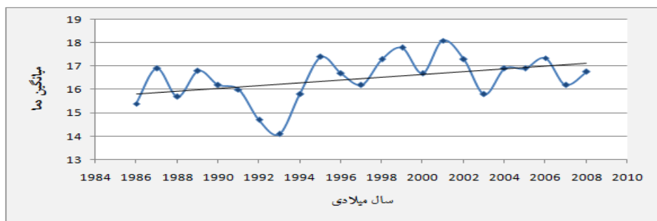
شکل ۸: نمودارهای روند میانگین دمای سالانه و نسبت بارش برف به بارش کل در ایستگاه خلخال
