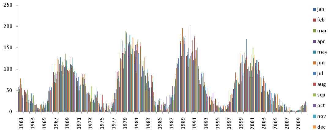
شکل ۴- تغییرات زمانی لکه‌های خورشیدی طی دوره آماری مورد مطالعه
