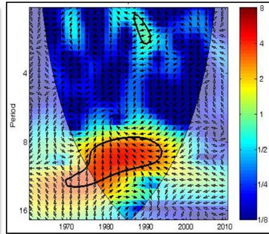
شکل ۵- تحلیل موجک پیوسته ماه فوریه
