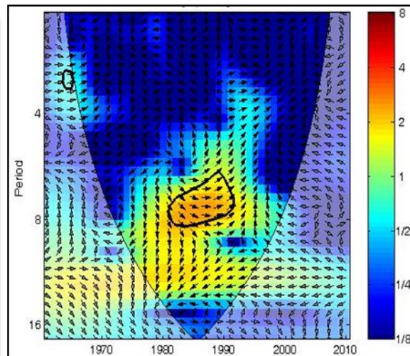
شکل ۱۳- تحلیل موجک پیوسته ماه آگوست
